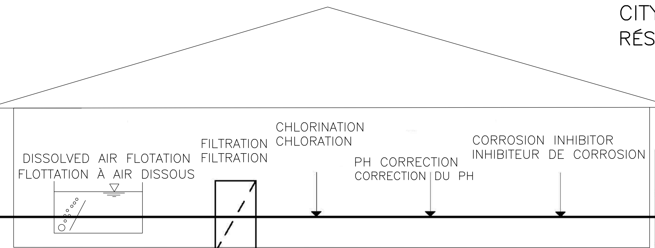
NEW WATER TREATMENT PLANT NOUVELLE USINE DE TRAITEMENT DES EAUX
